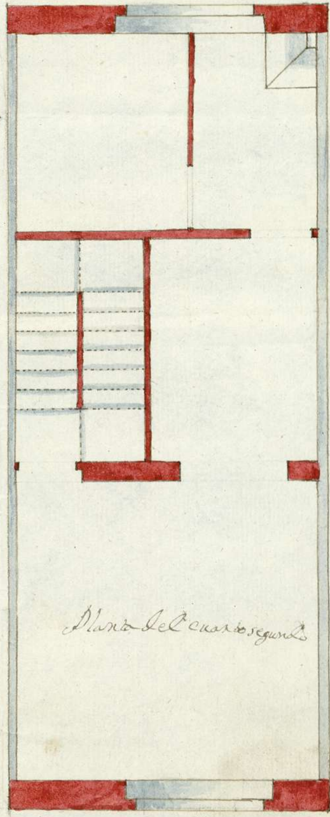
Planta del cuarto principal
